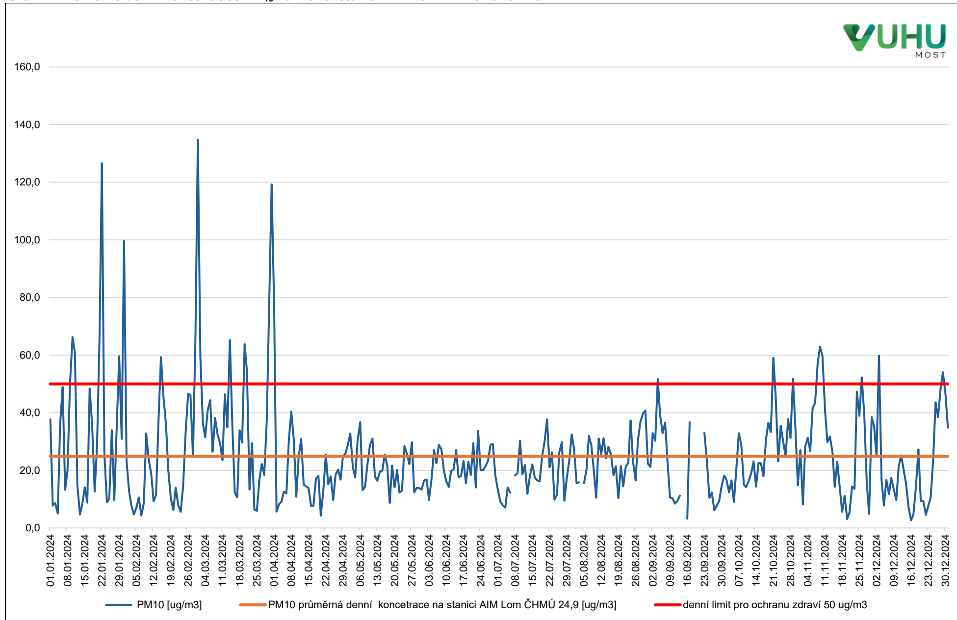
Graf 11: Průměrné denní koncentrace PM 10 na měřicí stanici AIM Lom ČHMÚ za rok 2024
