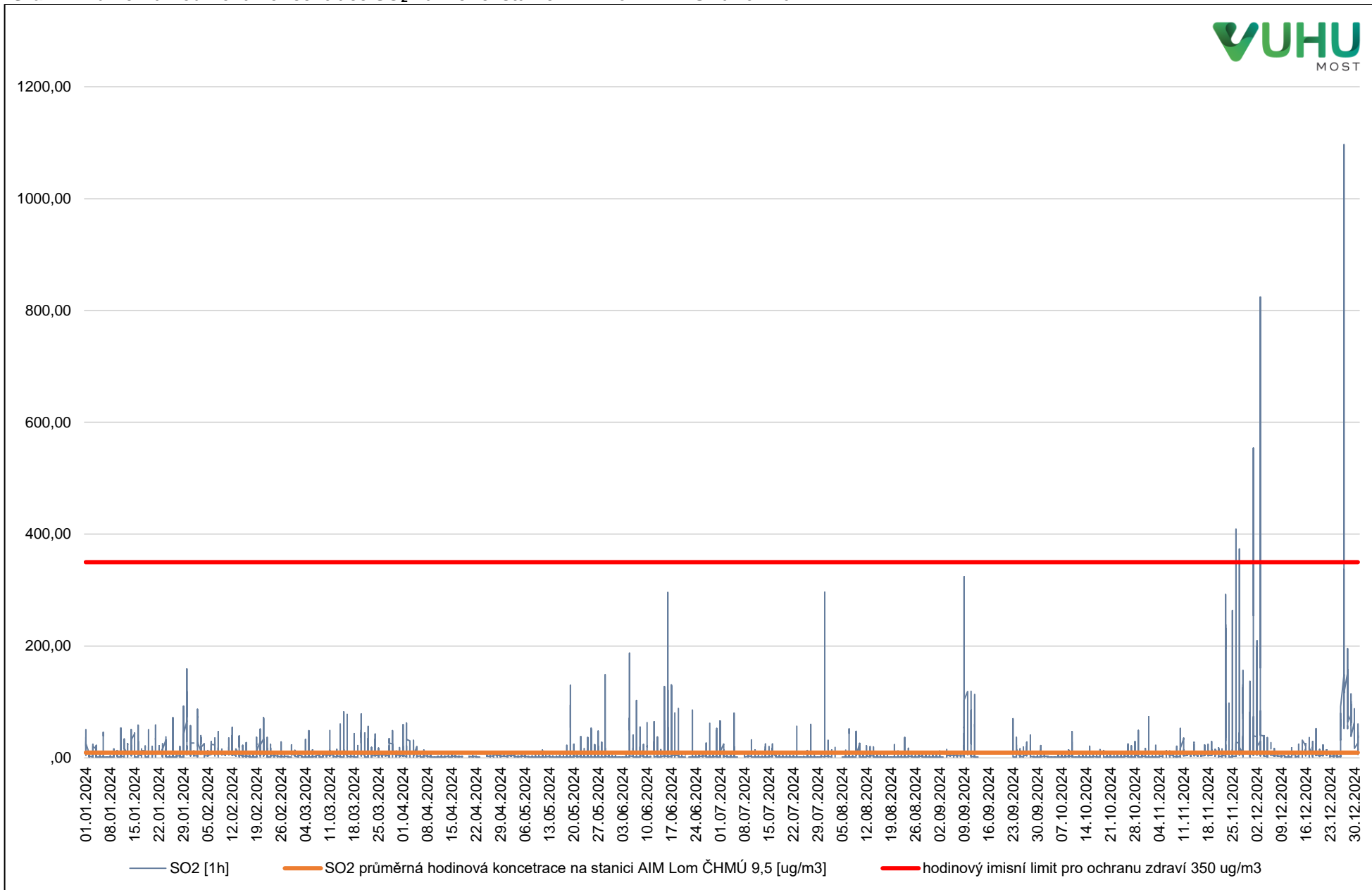
Graf 4: Průměrná hodinová koncentrace SO 2 na měřicí stanici AIM Lom ČHMÚ za rok 2024
