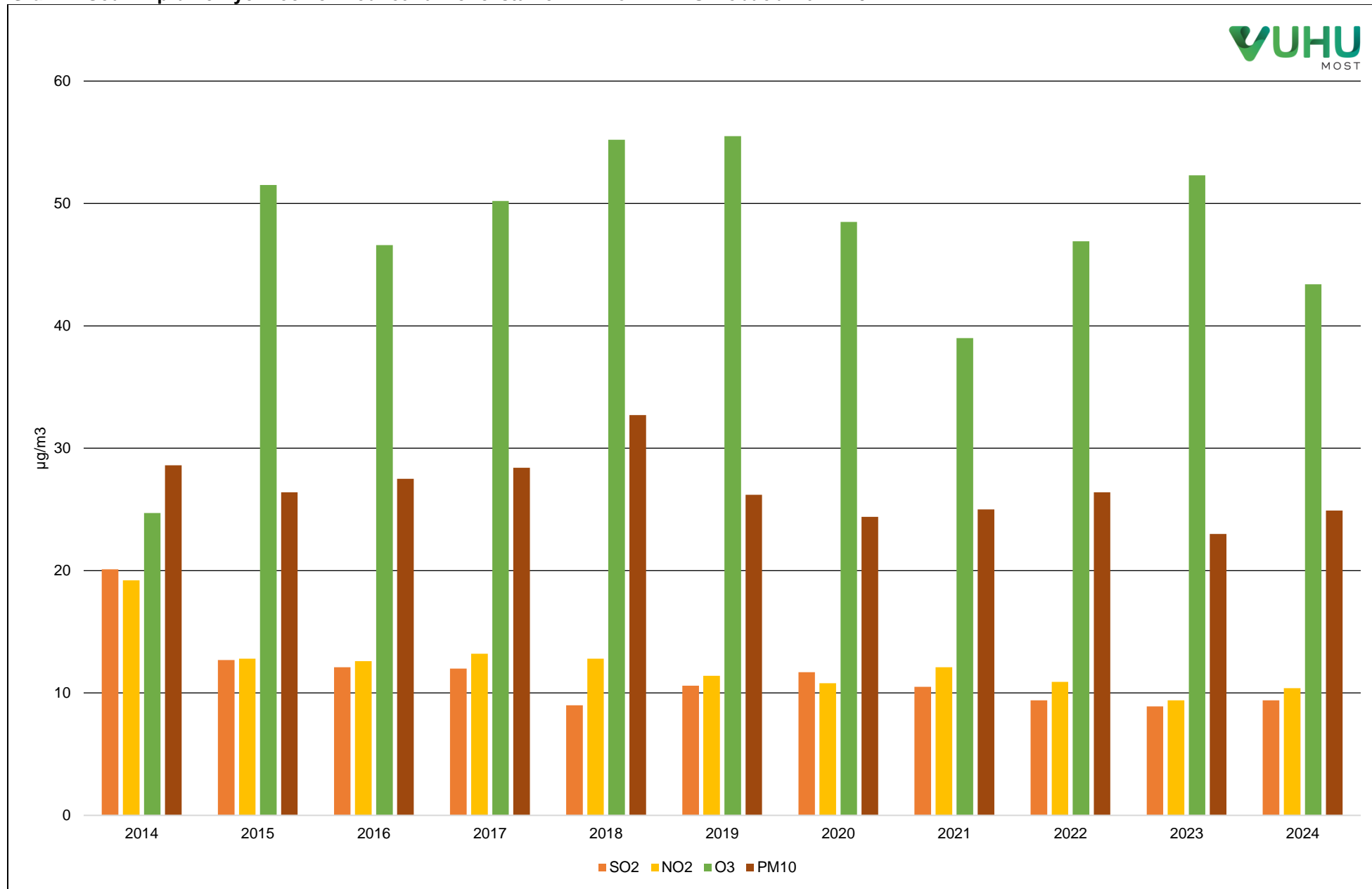
Graf 14: Souhrn průměrných ročních hodnot na měřicí stanici AIM Lom ČHMÚ v období 2014–2024
