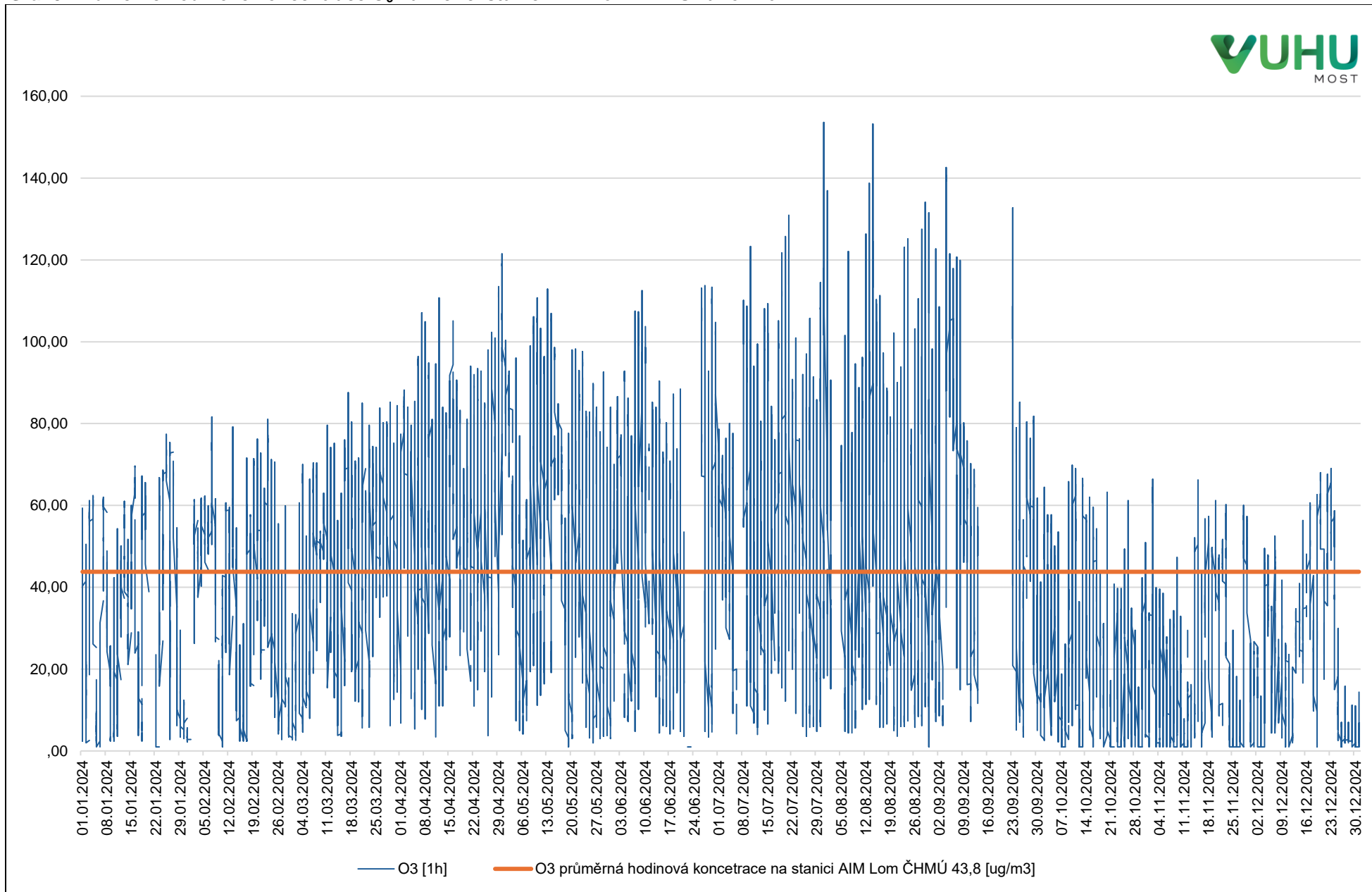
Graf 8: Průměrné hodinové koncentrace O 3 na měřící stanici AIM Lom ČHMÚ za rok 2024
