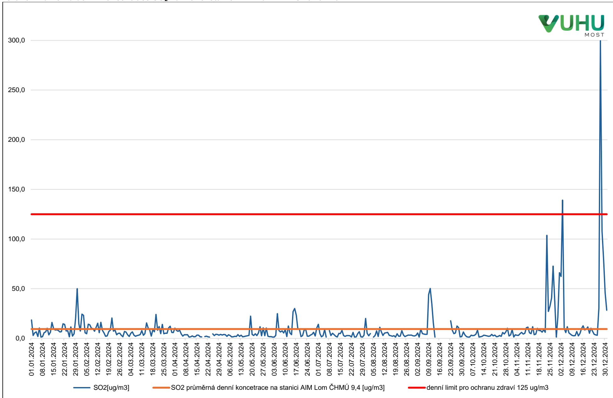
Graf 5: Průměrná denní koncentrace SO 2 na měřicí stanici AIM Lom ČHMÚ za rok 2024
