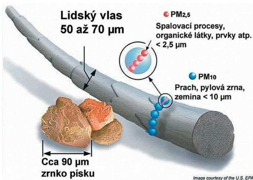
Obrázek 9: Poléťavý prach PM 10 , PM 2,5
