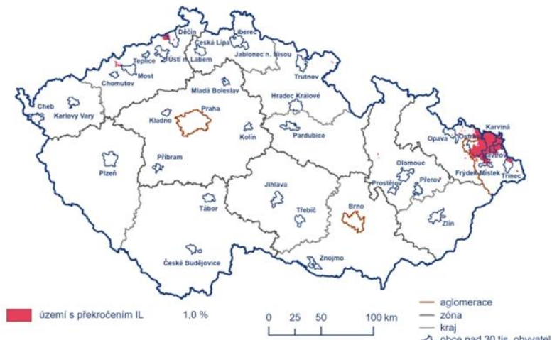
Obrázek 4: Překročení imisních limitů pro ochranu zdraví lidí pro rok 2023 v celé ČR bez zahrnutí přízemního ozonu
