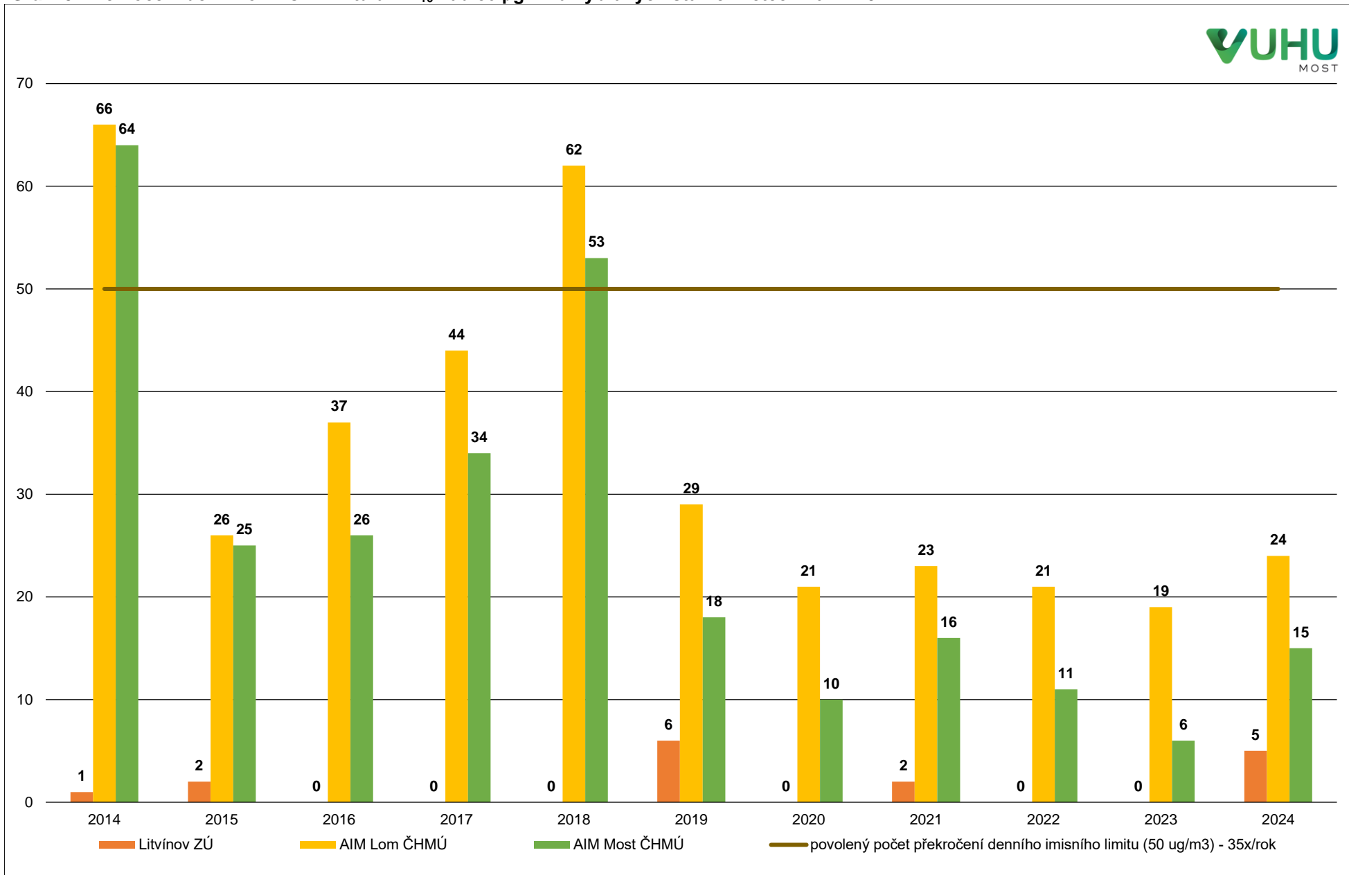
Graf 15: Překročení denního imisní limitu u PM 10 nad 50 µg/m 3 u vybraných stanic v letech 2014–2024
