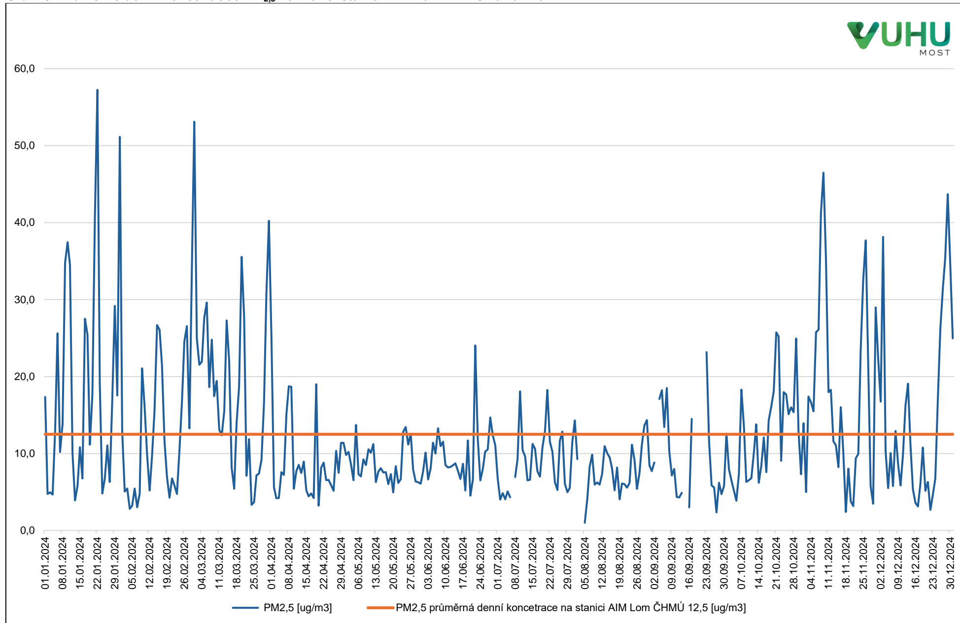
Graf 13: Průměrné denní koncentrace PM 2,5 na měřicí stanici AIM Lom ČHMÚ za rok 2024
