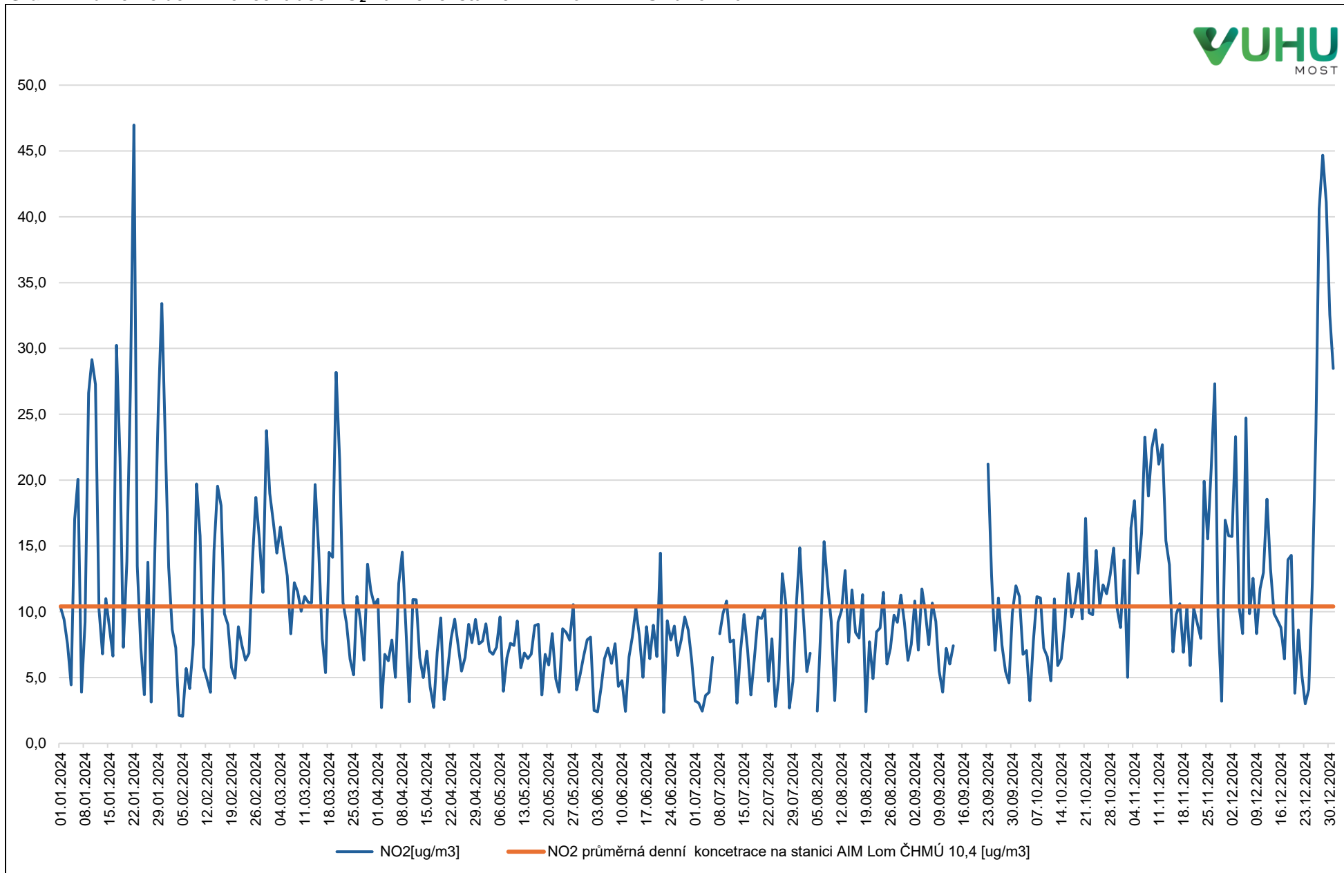
Graf 7: Průměrné denní koncentrace NO 2 na měřicí stanici AIM Lom ČHMÚ za rok 2024
