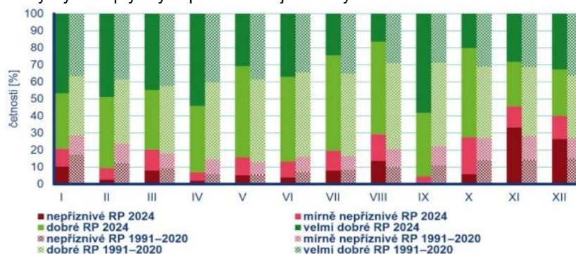
Obrázek 2: Četnosti výskytu rozptylových podmínek v jednotlivých měsících
