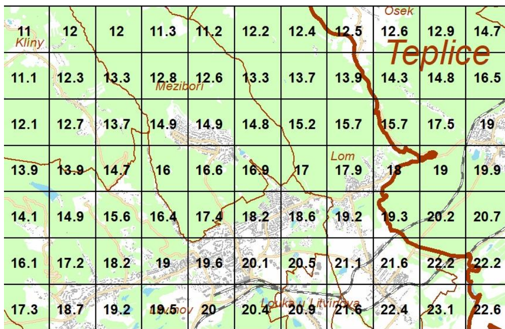
Obrázek 5: Pětiletá průměrná koncentrace částic PM 10 na Litvínovsku r. 2019–2023
