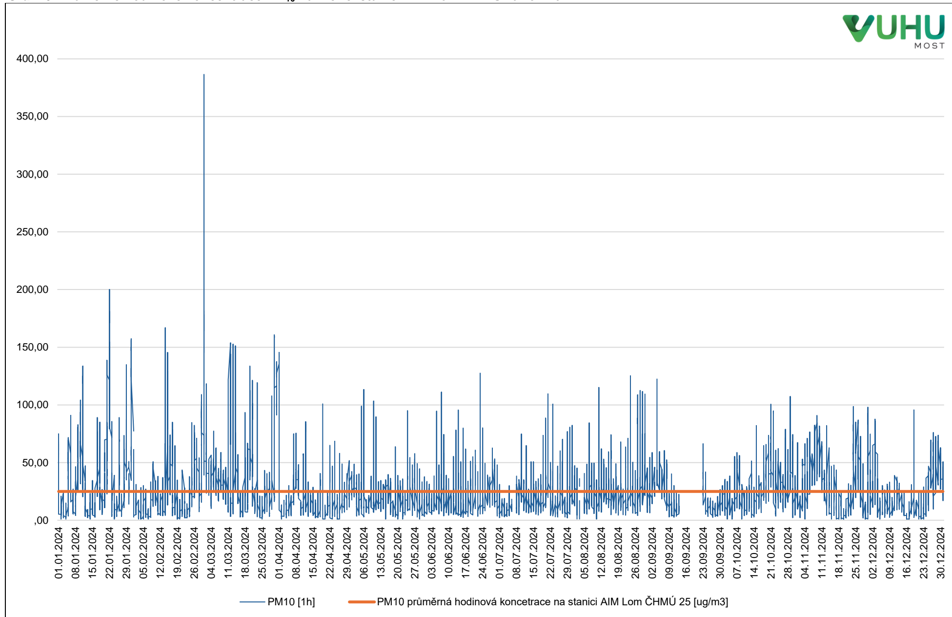
Graf 10: Průměrné hodinové koncentrace PM 10 na měřicí stanici AIM Lom ČHMÚ za rok 2024
