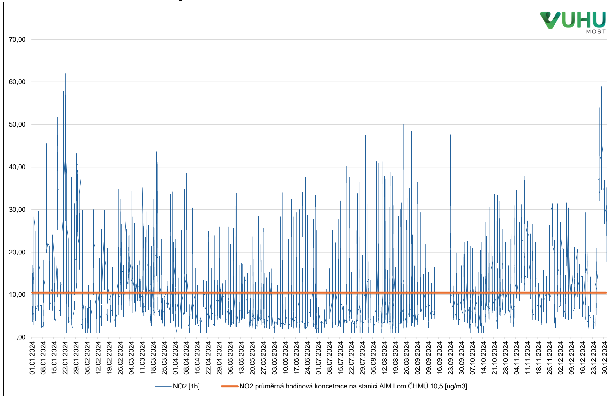
Graf 6: Průměrné hodinové koncentrace NO 2 na měřicí stanici AIM Lom ČHMÚ za rok 2024
