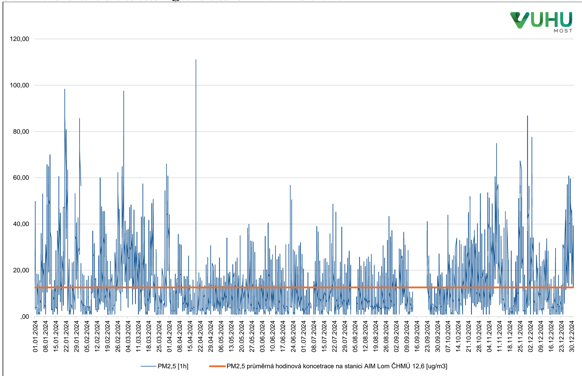
Graf 12: Průměrné hodinové koncentrace PM_{2,5} na měřicí stanici AIM Lom ČHMÚ za rok 2024
