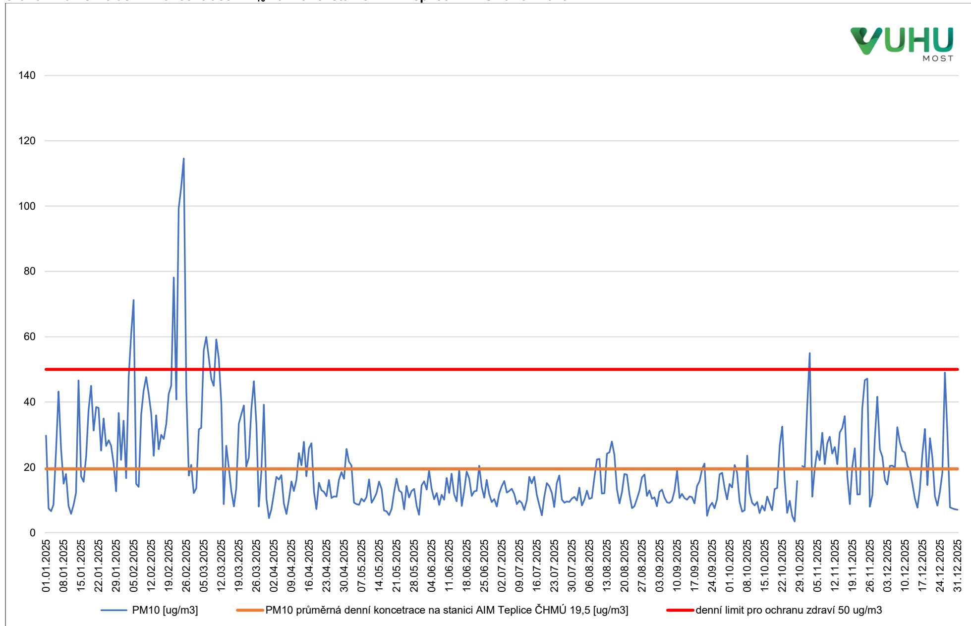
Graf 9: Průměrné denní koncentrace PM 10 na měřicí stanici AIM Teplice ČHMÚ za rok 2025
