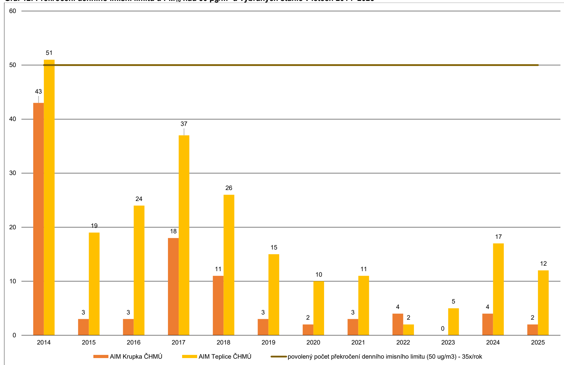
Graf 12: Překročení denního imisní limitu u PM 10 nad 50 µg/m 3 u vybraných stanic v letech 2014–2025
