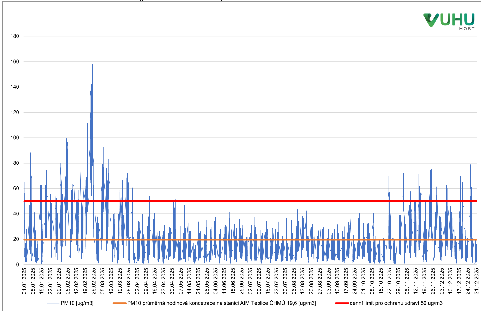
Graf 8: Průměrné hodinové koncentrace PM 10 na měřicí stanici AIM Teplice ČHMÚ za rok 2025
