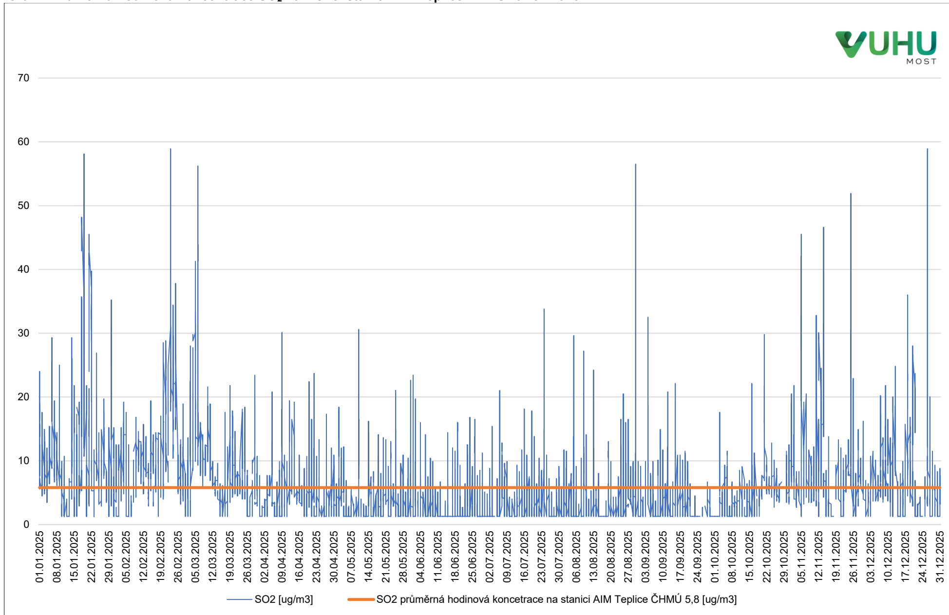
Graf 4: Průměrná hodinová koncentrace SO 2 na měřicí stanici AIM Teplice ČHMÚ za rok 2025
