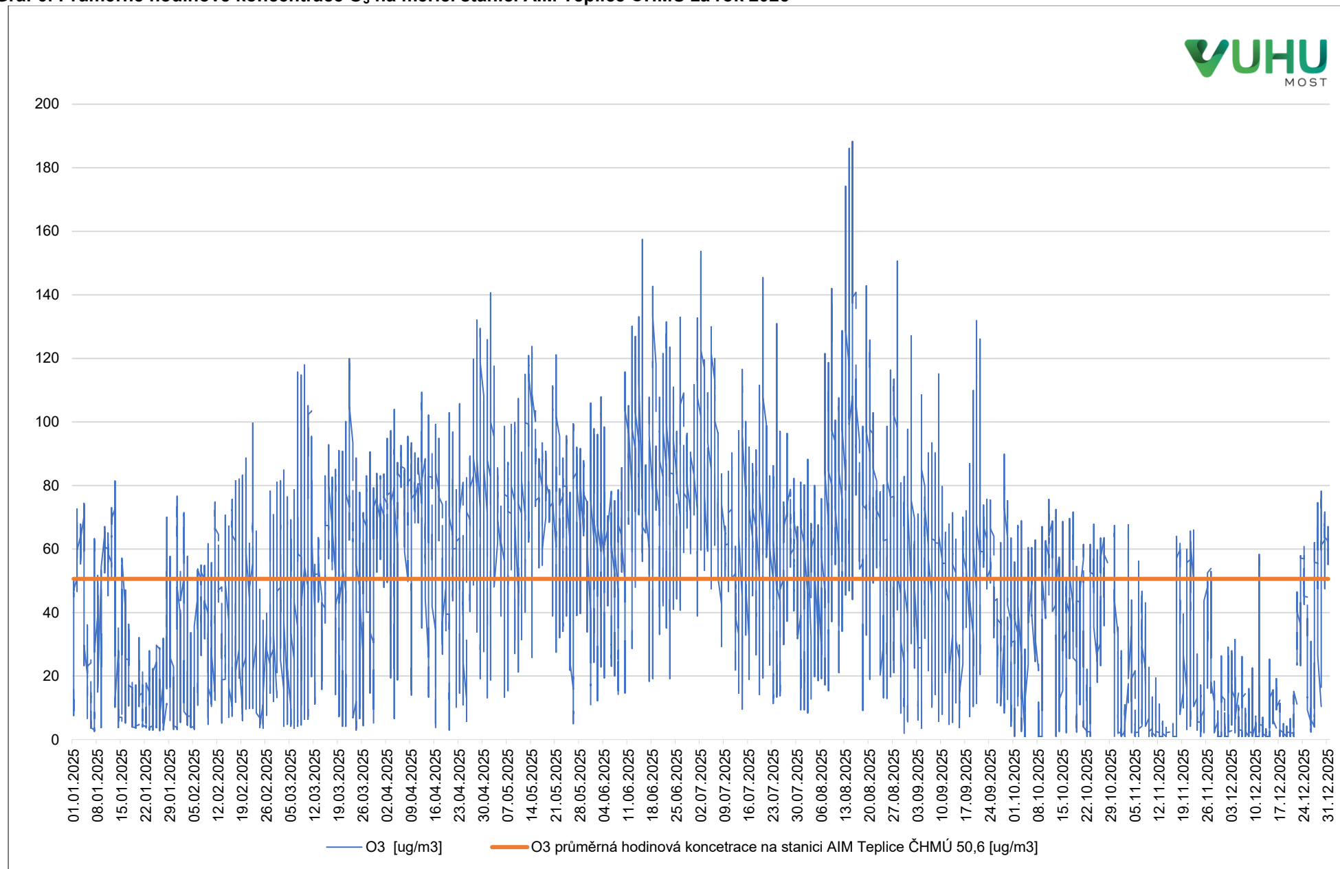
Graf 6: Průměrné hodinové koncentrace O 3 na měřicí stanici AIM Teplice ČHMÚ za rok 2025
