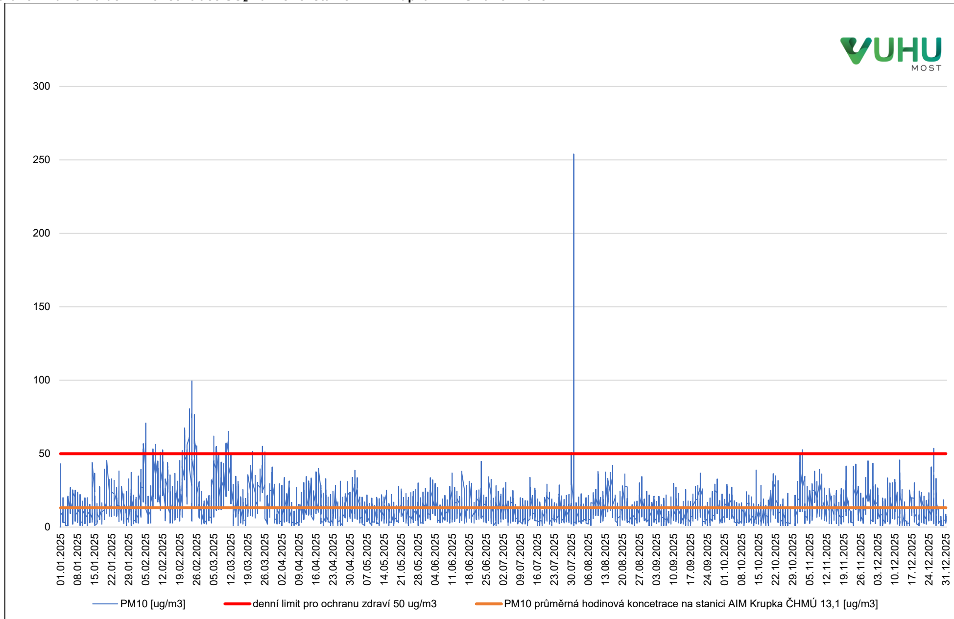
Graf 5: Průměrná denní koncentrace SO 2 na měřicí stanici AIM Krupka ČHMÚ za rok 2025
