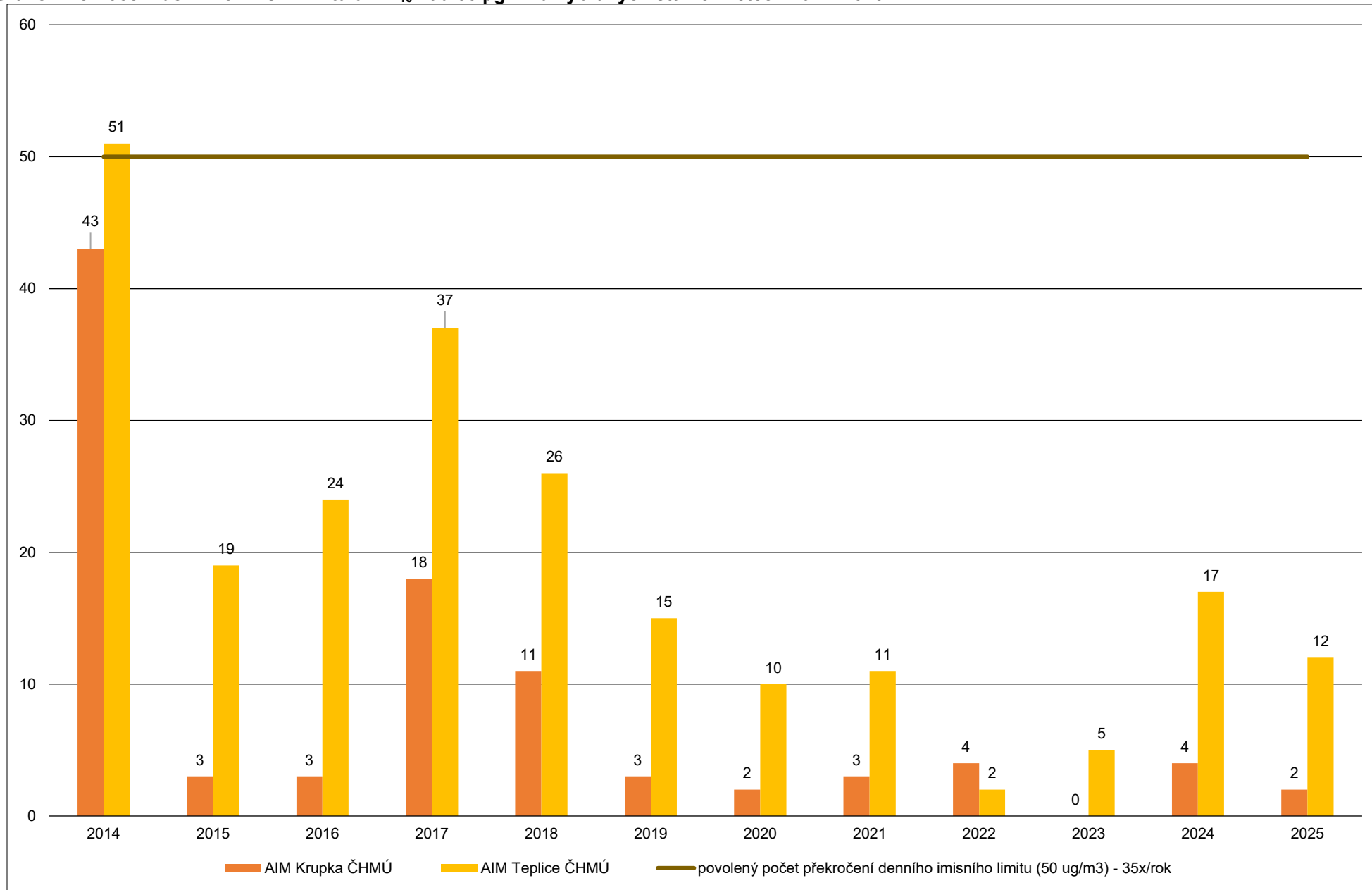
Graf 8: Překročení denního imisní limitu u PM 10 nad 50 µg/m 3 u vybraných stanic v letech 2014–2025
