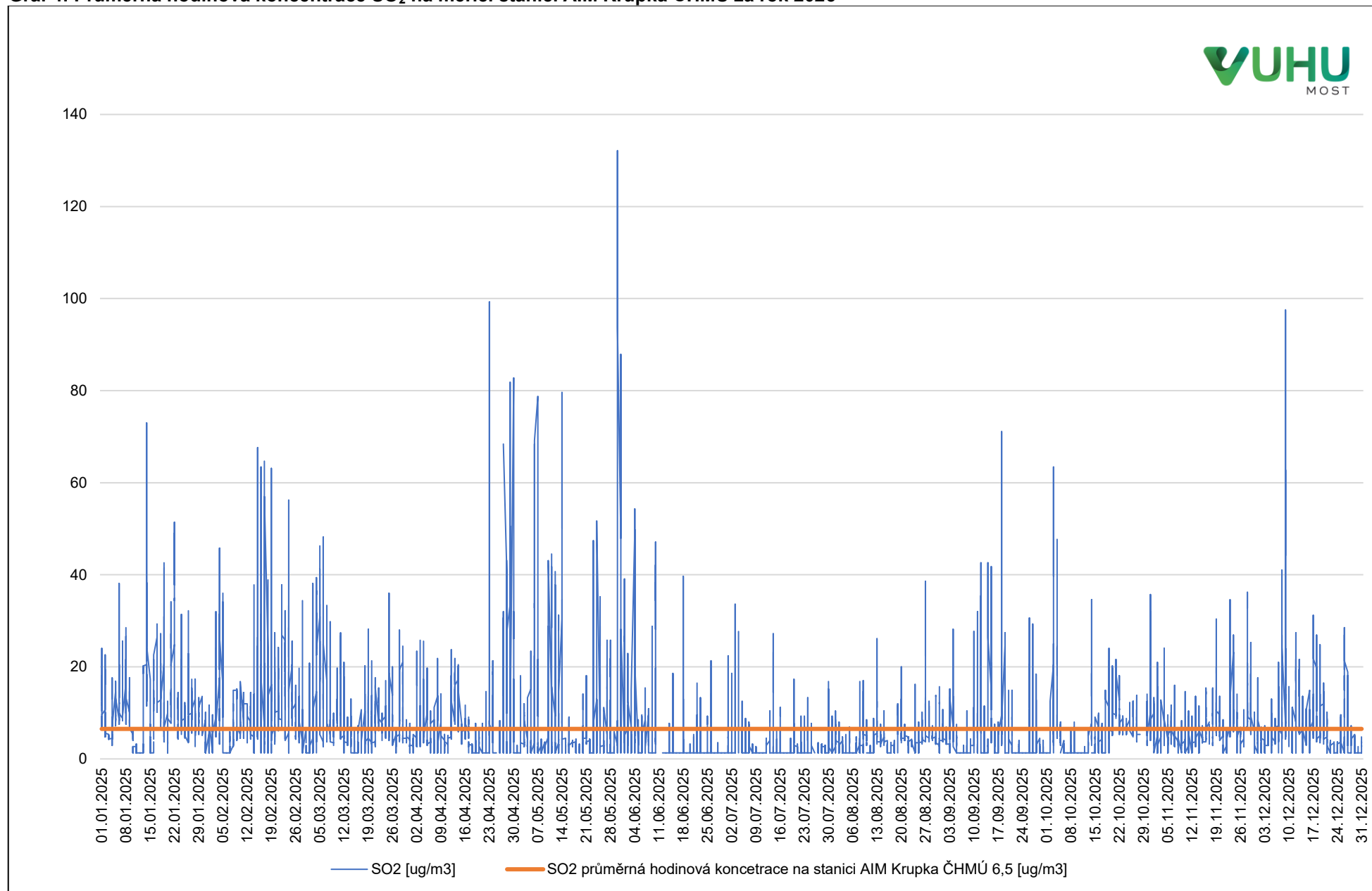
Graf 4: Průměrná hodinová koncentrace SO 2 na měřicí stanici AIM Krupka ČHMÚ za rok 2025
