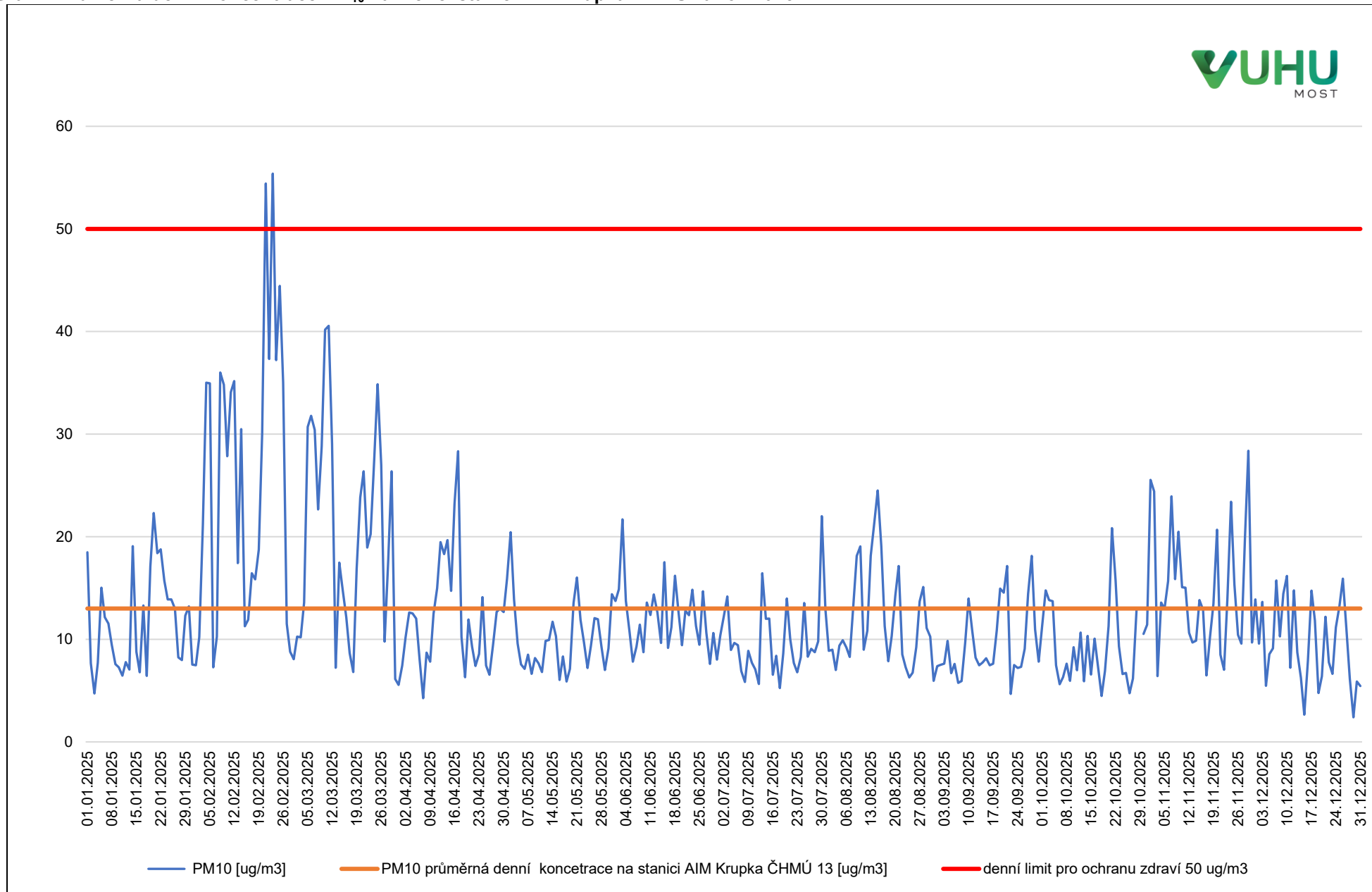
Graf 7: Průměrná denní koncentrace PM 10 na měřicí stanici AIM Krupka ČHMÚ za rok 2025
