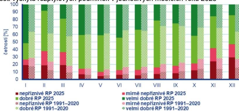
Obrázek 2: Četnosti výskytu rozptylových podmínek v jednotlivých měsících roku 2025
