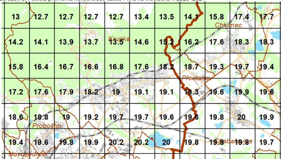
Obrázek 5: Pětiletá průměrná koncentrace částic PM 10 na Mostecku r. 2020–2024
