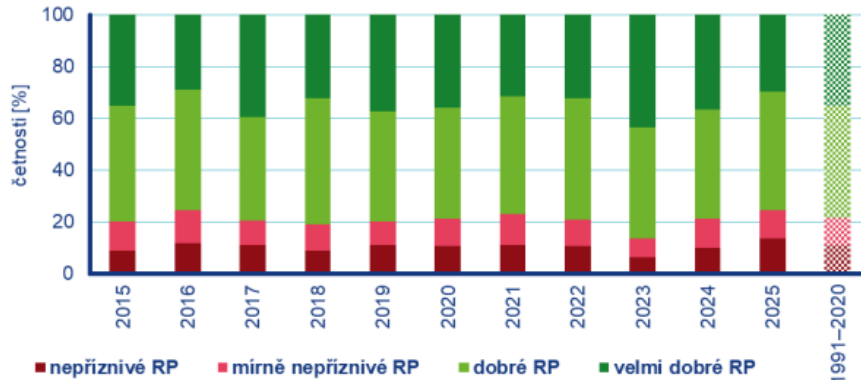
Obrázek 1: Četnosti výskytu rozptylových podmínek, 2015-2025
